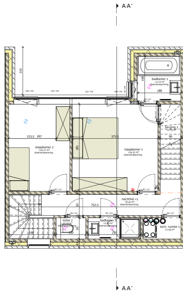
VERDIEPING 1 - 57,37 m 2
