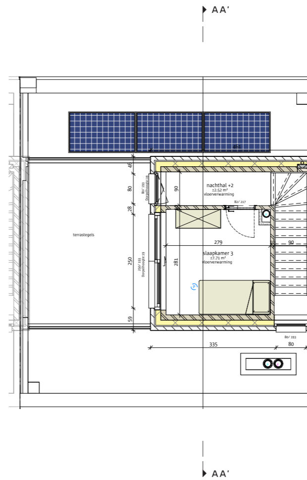
VERDIEPING 2 - 21,34 m 2
