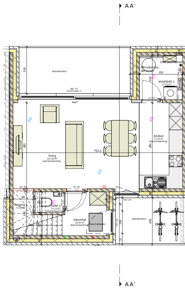
GELIJKVLOERS - 51,44 m 2
