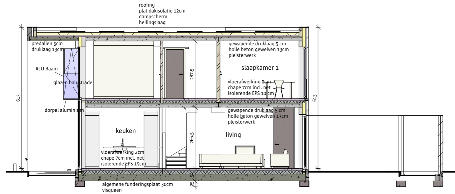
SNEDE AA'
